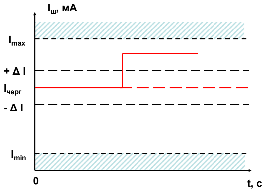
Рис. 2 – Часова діаграма зміни струму в шлейфі сигналізації: I_{\text{чєрг}} – струм шлейфу в черговому режимі; I_{\text{max}} – струм короткого замкнення; I_{\text{min}} – струм обриву шлейфу; \Delta I – порогове значення струму шлейфу при спрацьовуванні пожежного сповіщувача.
